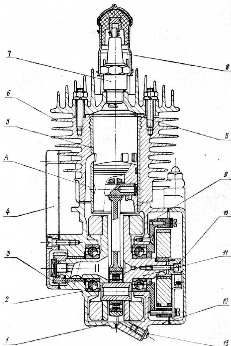
Рис. 2. Разрез двигателя:
