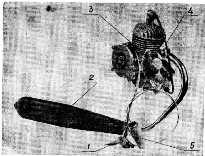
Рис. 1. Двигатель Д8:
