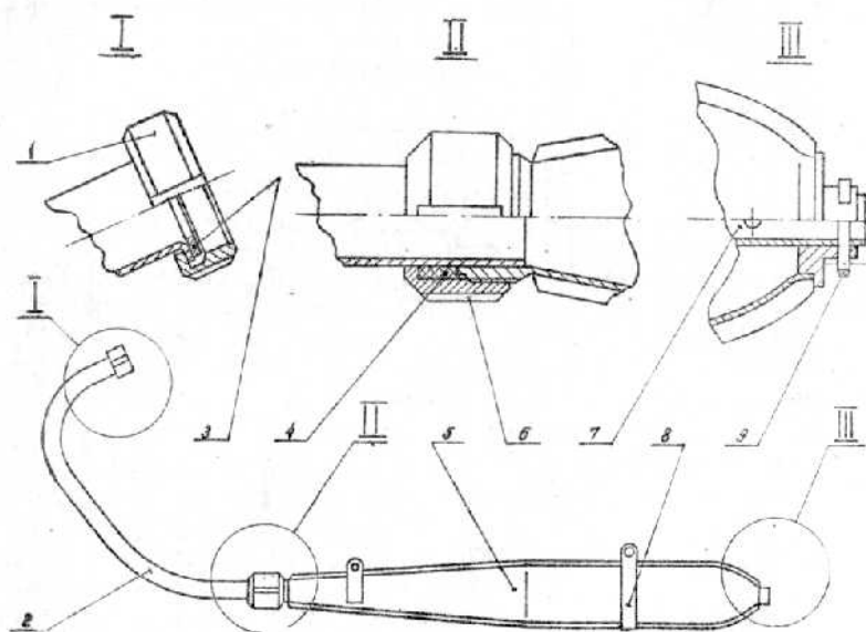
Рис. 7. Глушитель:
