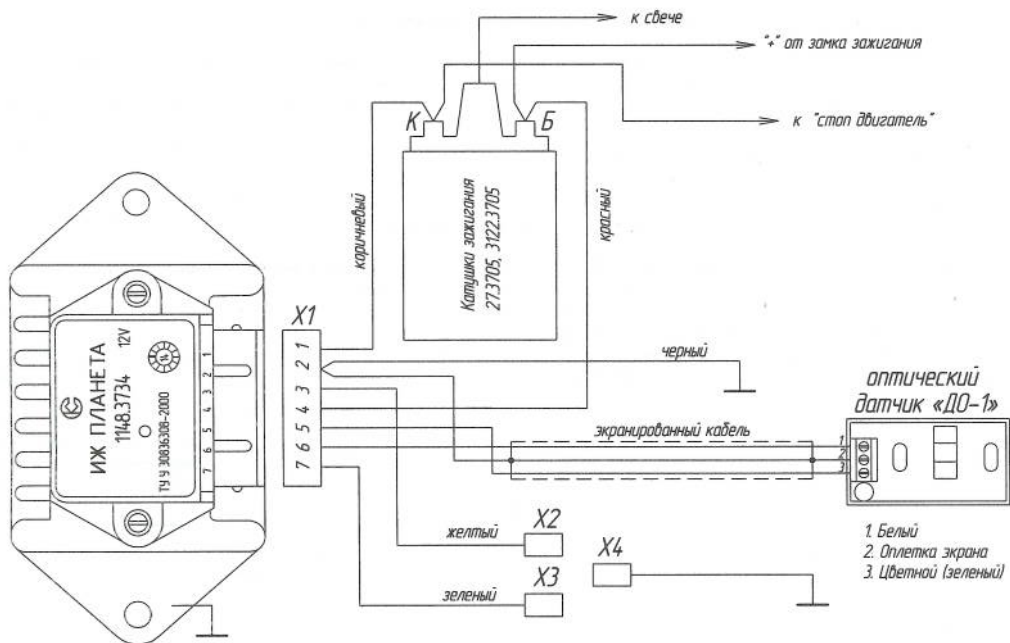
Рис.2. Схема установки МПБСЗ на мотоциклы с катушками 3122.3705 или 27.3705.
